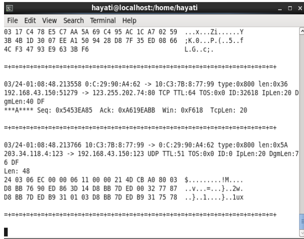
Gambar 9. Aktivitas Sistem
